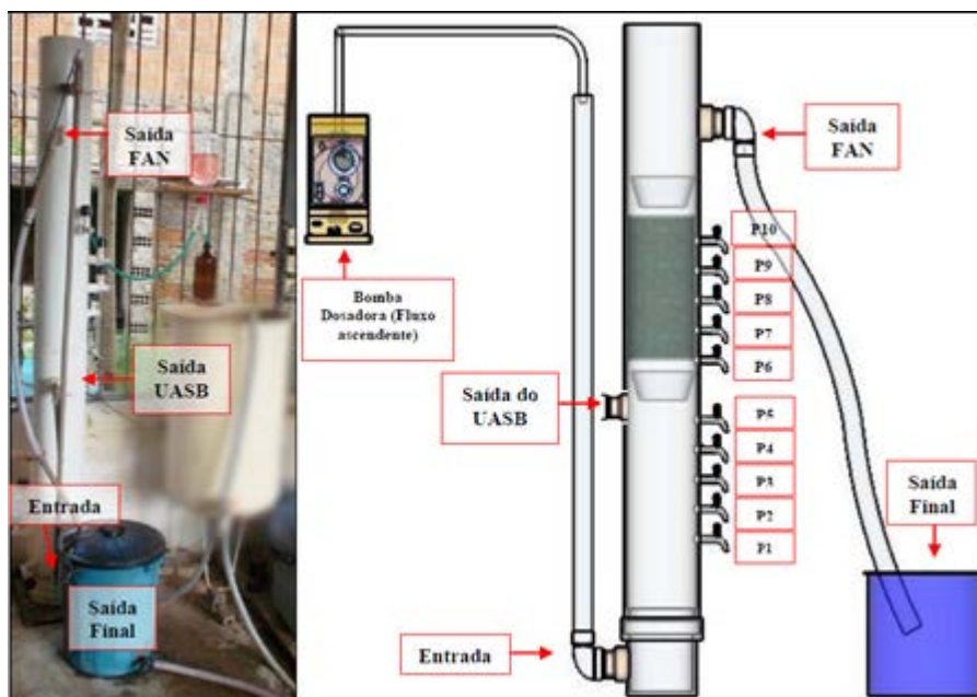
Figura 1: Reator Anaeróbio Híbrido – RAH. Fonte: Lima, 2015.
