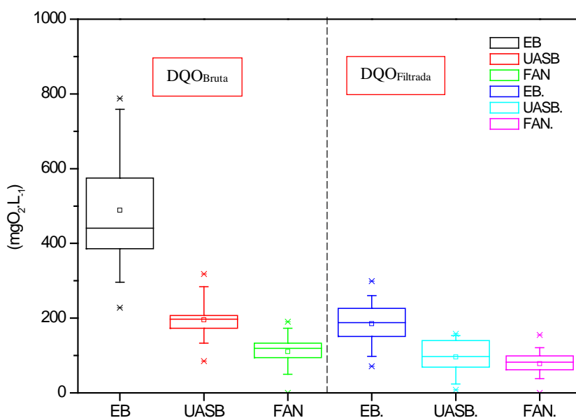
Figura 2: Comportamento de material carbonáceo no RAH.
