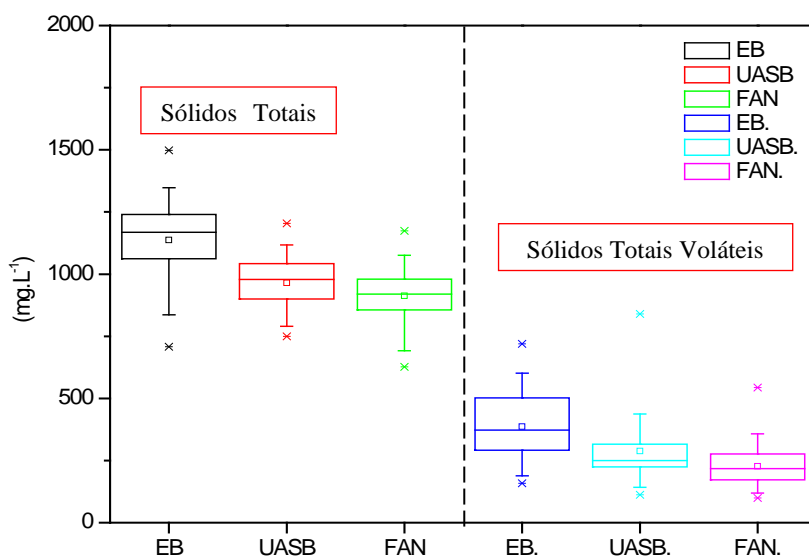
Figura 3: Comportamento dos sólidos totais e dos sólidos totais voláteis no RAH.
