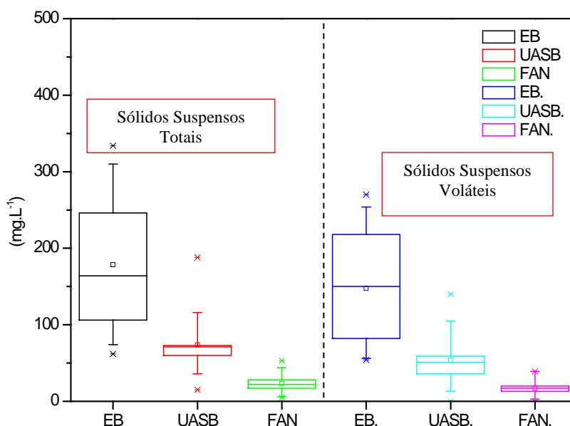
Figura 4: Comportamento dos sólidos suspensos totais e dos sólidos suspensos voláteis no RAH.
